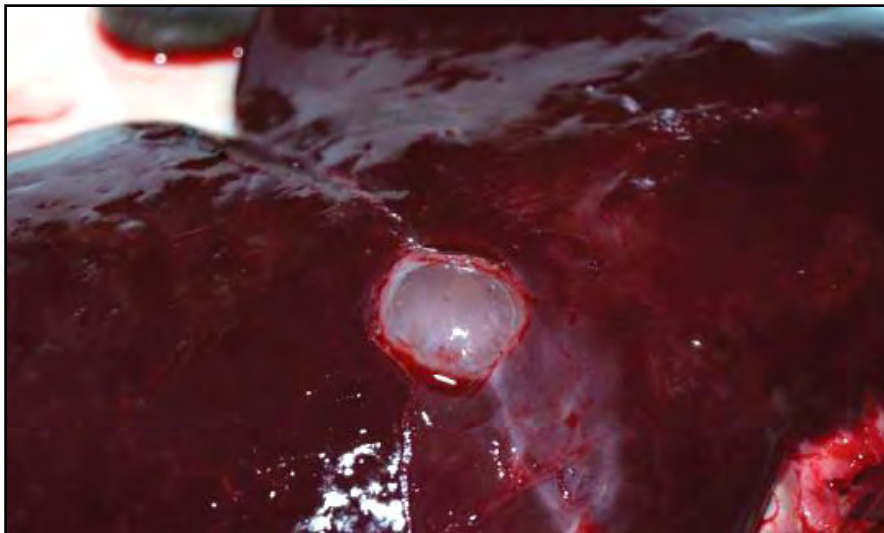
Figura 11.- Cysticercus ovis .
